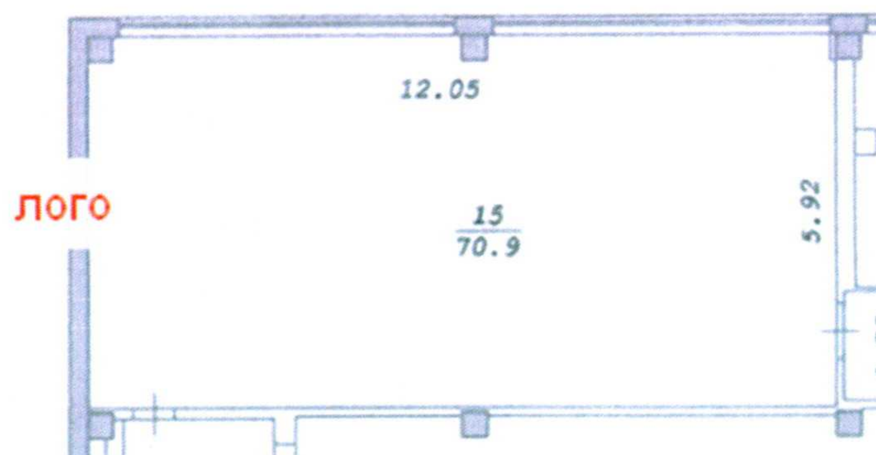
WEB-куб. План
